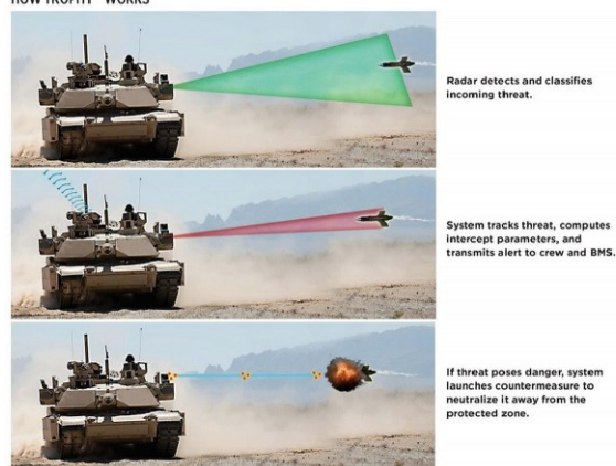
Způsob fungování systému Trophy
